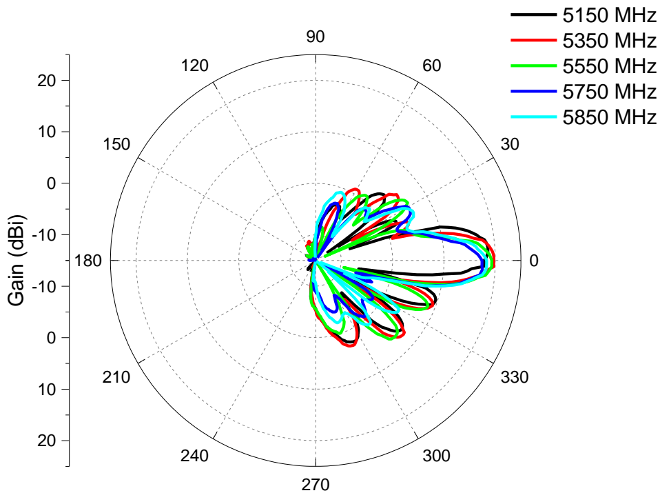
H-Plane -02
